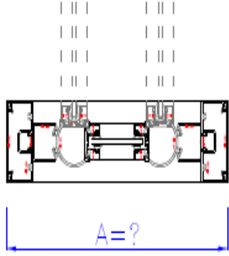
OPTION 3 DOUBLE DOOR SET
