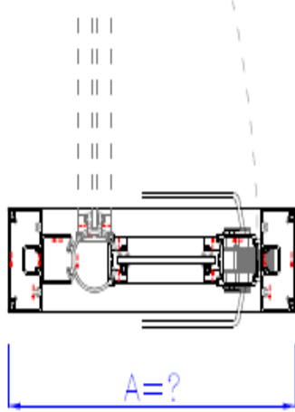
OPTION 2 SINGLE DOOR SET / FAN
