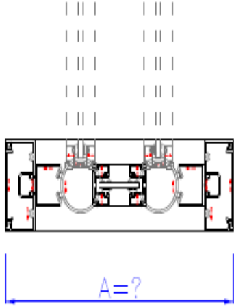
OPTION 4 DOUBLE DOOR SET/FAN
